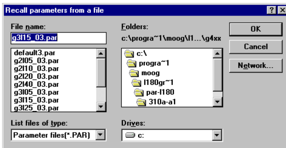
Figure 54: Parameter Download
