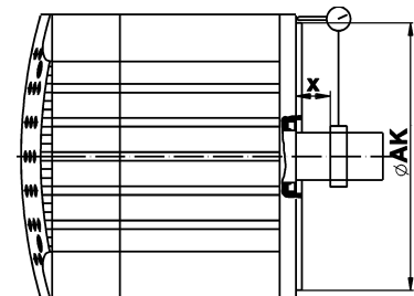
Planlauf / perpendicularity
