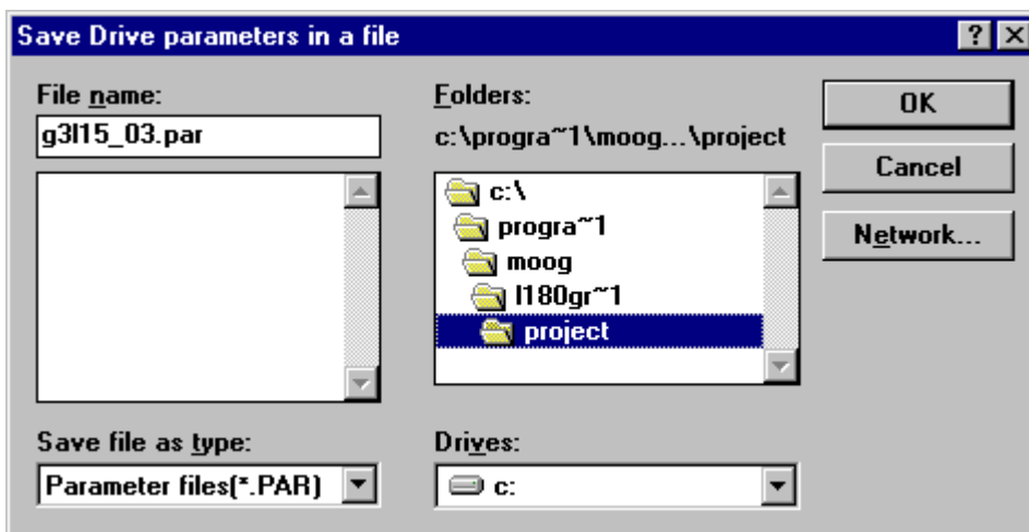
Figure 70: Parameter Upload
