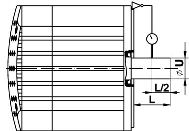
Rundlauf / runout
