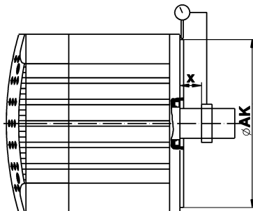
Koaxialität / concentricity
